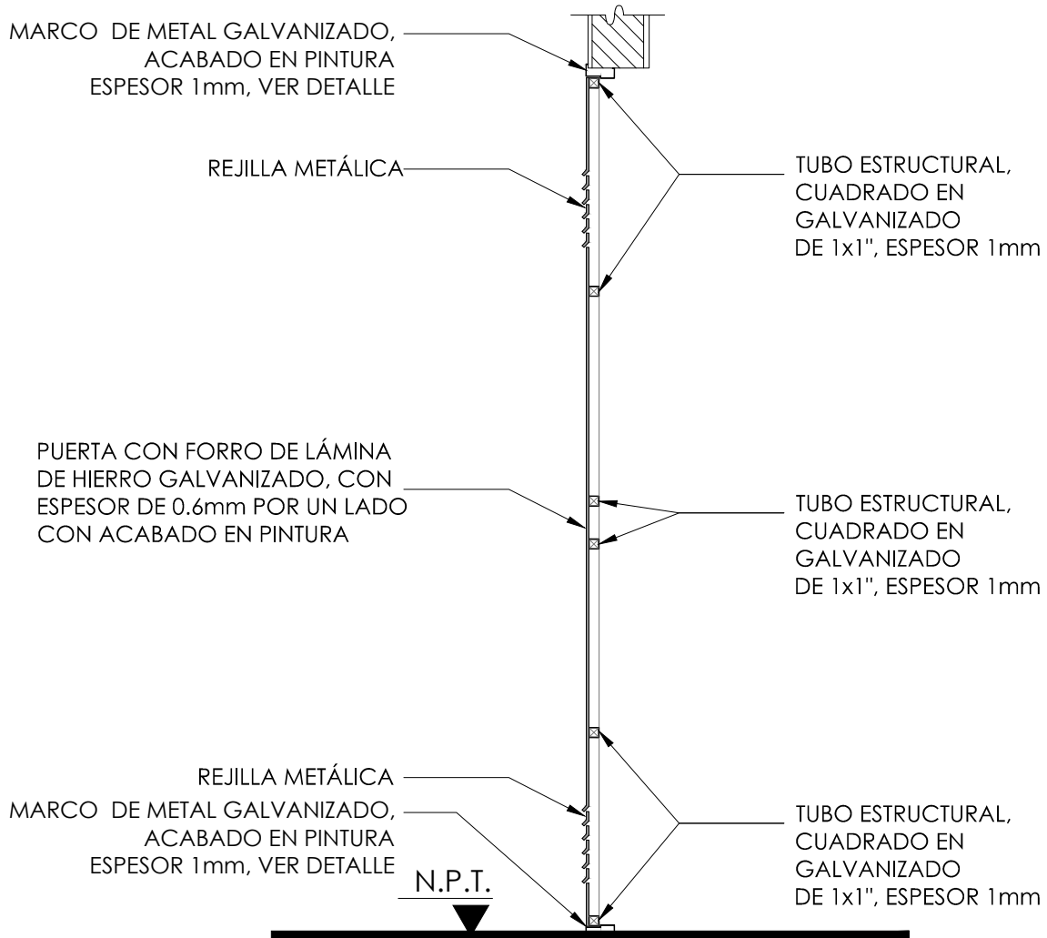
CORTE A-A
