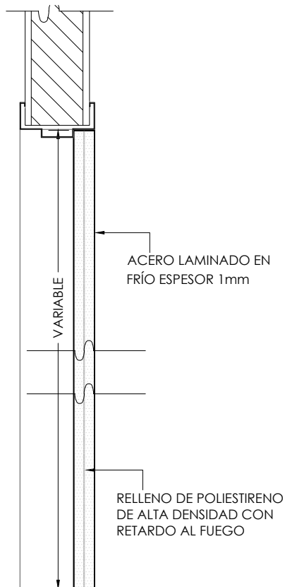
CORTE A-A
