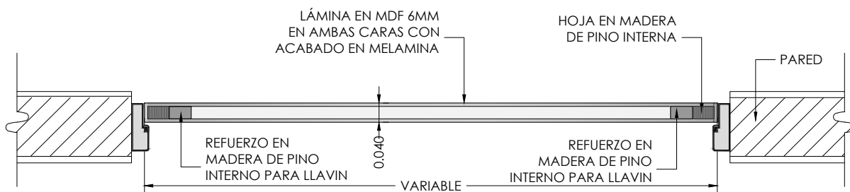
CORTE B-B
