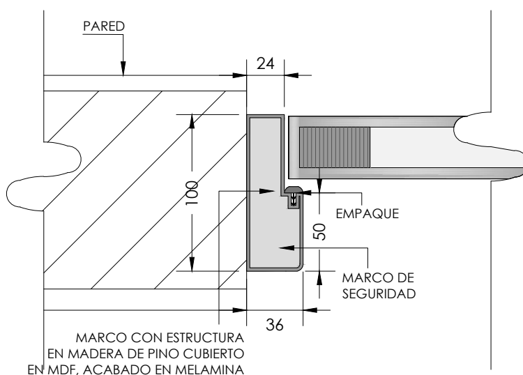
DETALLE MARCO
