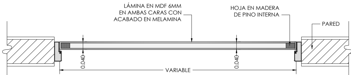
CORTE A-A
