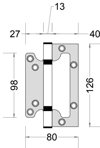
DETALLE BISAGRA TIPO MARIPOSA
