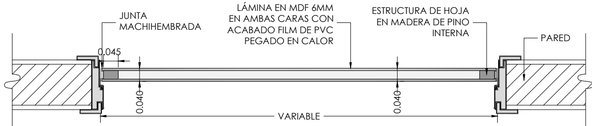
CORTE A-A
