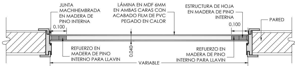
CORTE B-B
