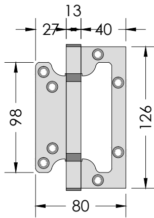
DETALLE BISAGRA TIPO MARIPOSA
