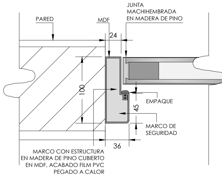
DETALLE MARCO
