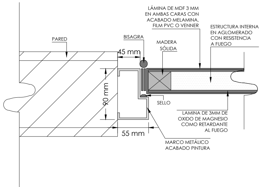
DETALLE MARCO
