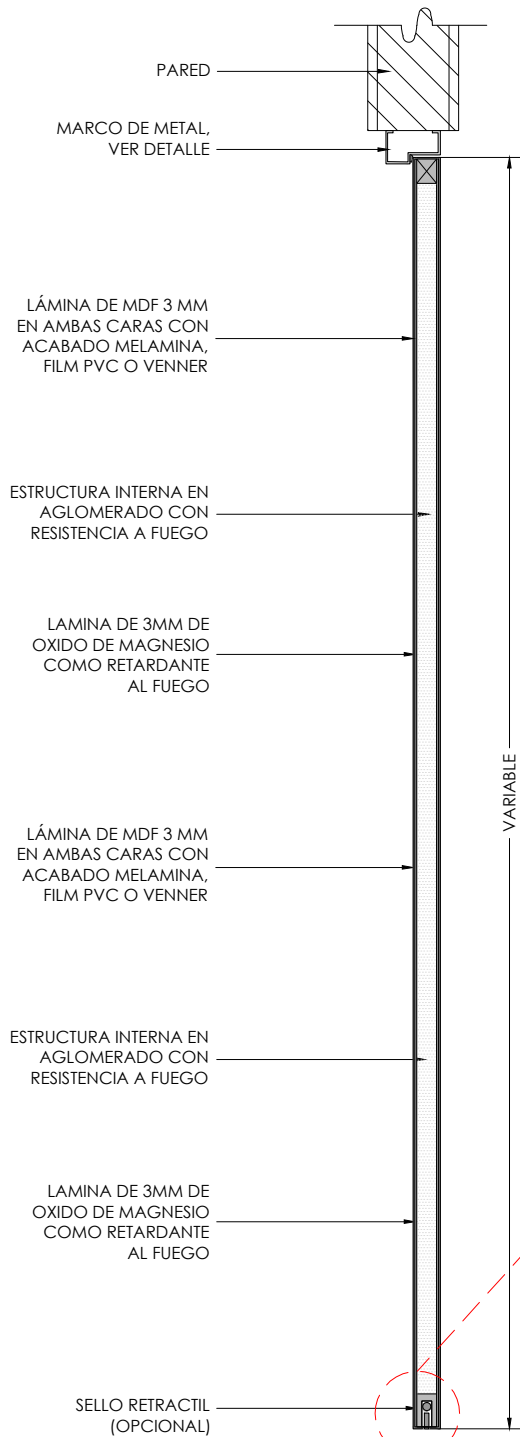
CORTE B-B
